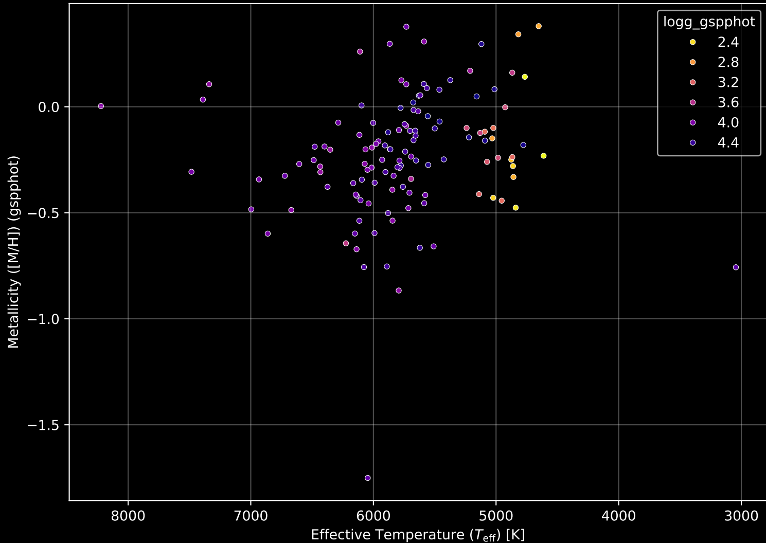
GALAH DR4 Field: [7180] Stellar Population Parameters (n= 126)
