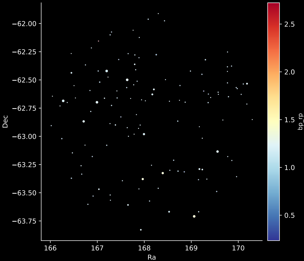
GALAH DR4 Field: [7180] Stars: 126
